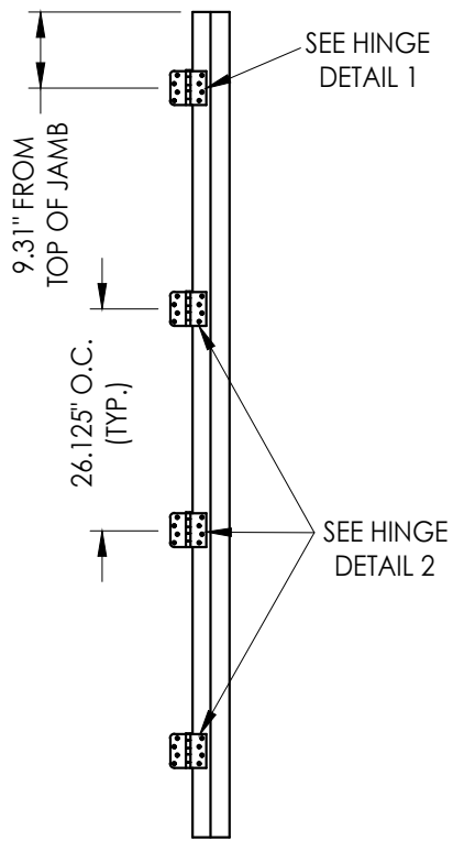
HINGE JAMB
