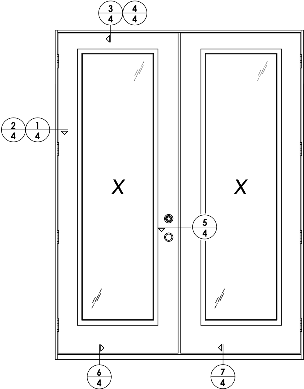
ELEVATION XX
